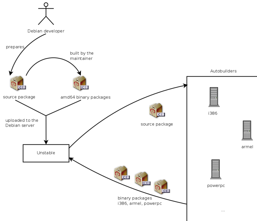
Figura 1.2 Compilación de un paquete por los autobuilders
