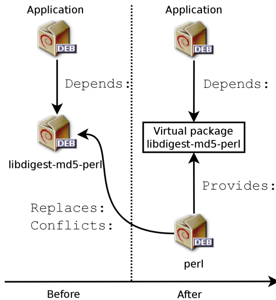
Figura 5.1 Utilización del campo Provides para no romper dependencias
