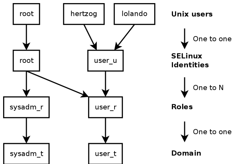
Figura 14.3 Contextos de seguridad y usuarios Unix
