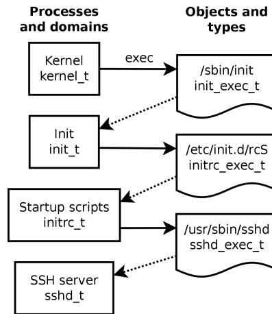
Figura 14.4 Transiciones automáticas entre dominios
